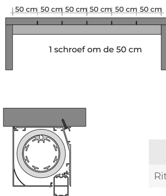
Montage op de pergola (schroeven)
